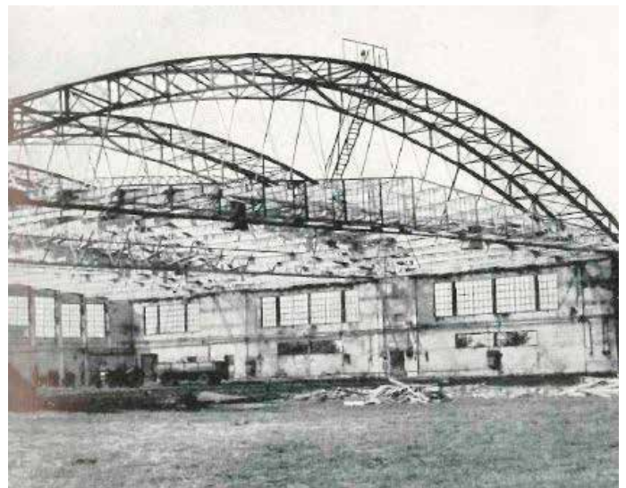
Uszkodzony hangar na lotnisku Rakowice. Fot. z archiwum autora
